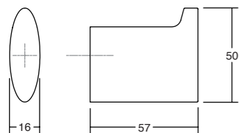
Fixation with screw Fijación con tornillo
