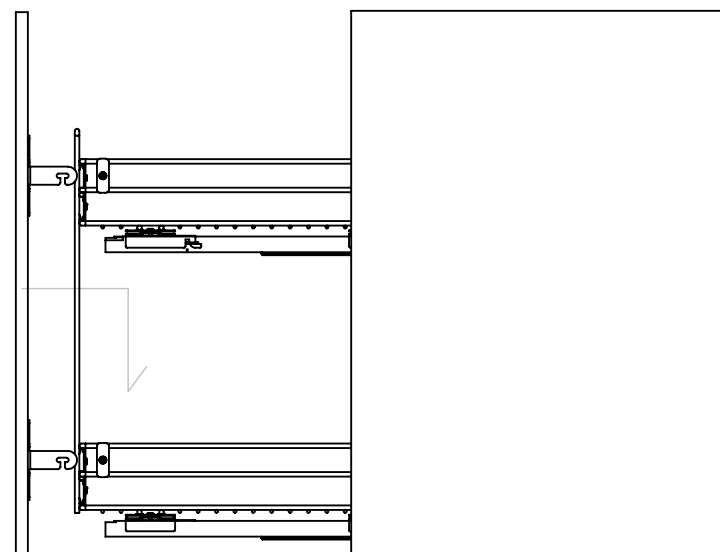
5. Установка и регулировка фасада
